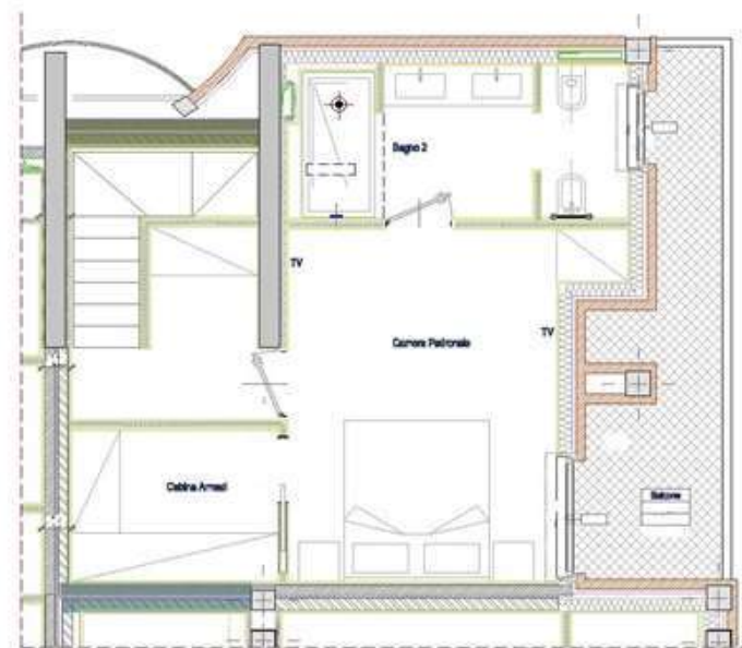
APPARTAMENTO 303 piano quarto layout architettonico
